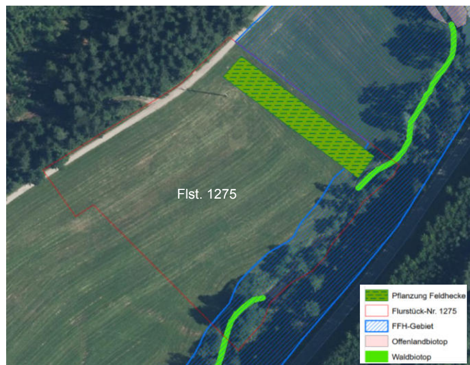
Abb. 1: Detaillage der Ausgleichsfläche (ca. 1230 qm) auf dem Flurstück 1275, Gemeinde Niedereschach.
